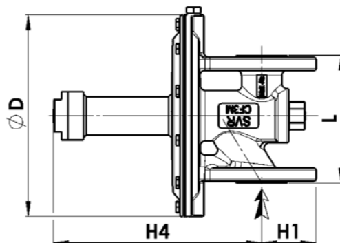
Déverseur piloté droit EPLP D
