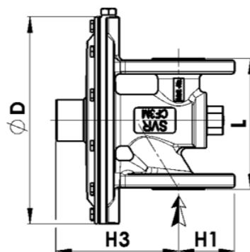
Déverseur cousin d'air droit EPLCA D
