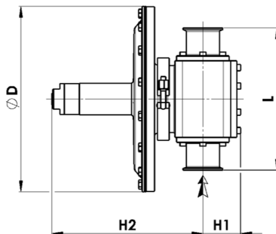
Déverseur droit Clean Clamp / Taraudé EPL D CL
