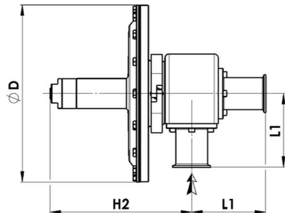
Déverseur équerre Clean Clamp / Taraudé EPL L CL
