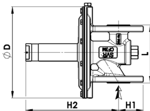
Déverseur droit EPL D
