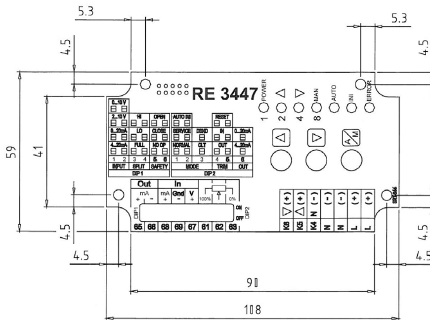
Dimension sheet / Encombrement
